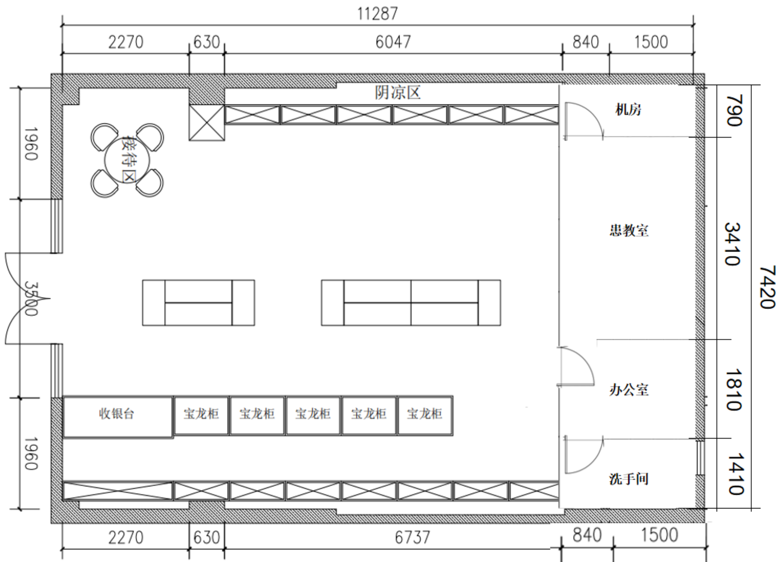
一层平面布置图
